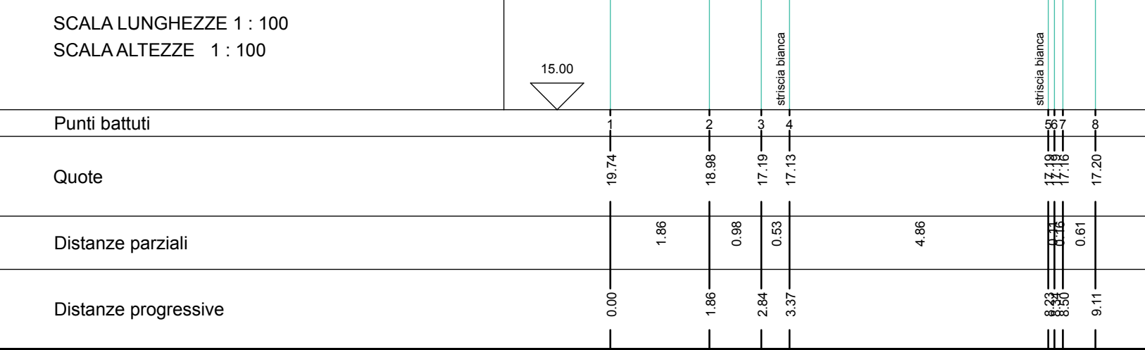
SEZIONE - 1 - STATO DI FATTO - Scala 1:100
