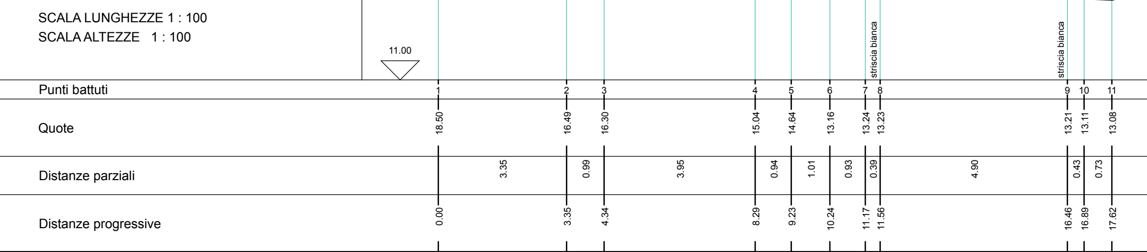
SEZIONE - 2 - STATO DI FATTO - Scala 1:100
