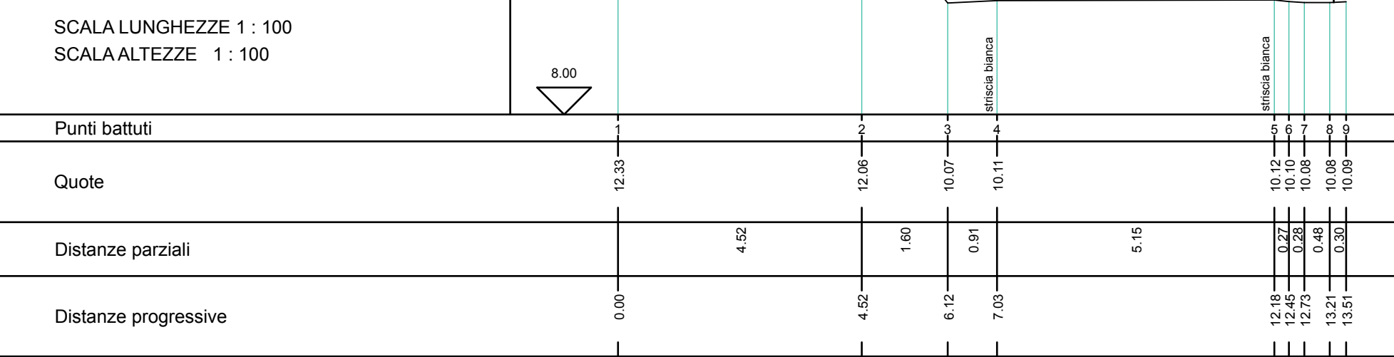
SEZIONE - 3 - STATO DI FATTO - Scala 1:100
